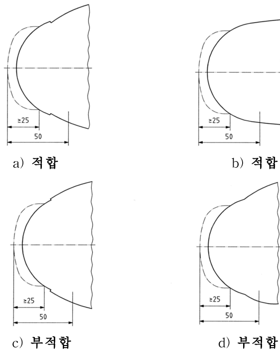
<그림 9> 자유 공간 2에서 축의 곡률의 보기
