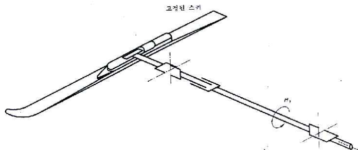
<그림 21> M_Y 토크의 적용 및 M_{Y,max} 측정
